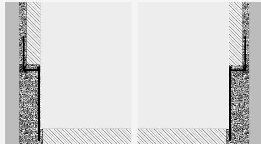
ESEMPI DI POSA - INSTALLATION EXAMPLES EXEMPLES DE POSE - VERLEGEBEISPIELE
