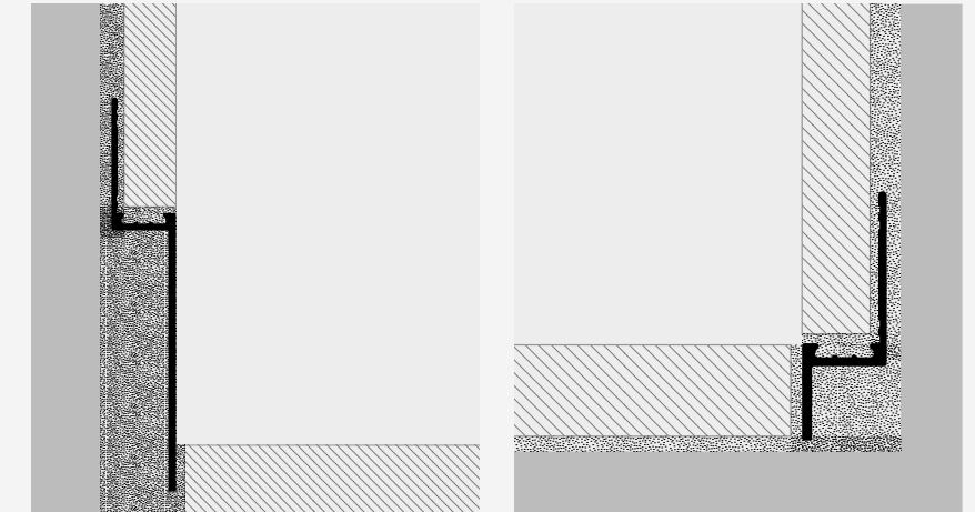
ESEMPI DI POSA - INSTALLATION EXAMPLES EXEMPLES DE POSE - VERLEGEBEISPIELE
